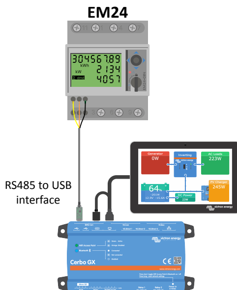
EM24 bekabelde verbinding met een Cerbo GX met behulp van een RS485-naar-USB-interface
