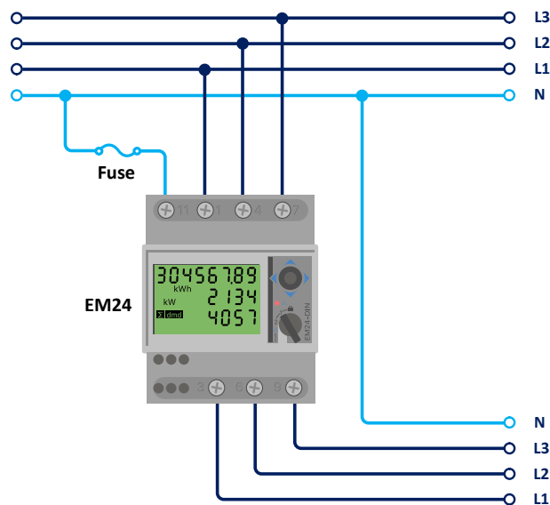
EM24-bedrading 3-fasen
