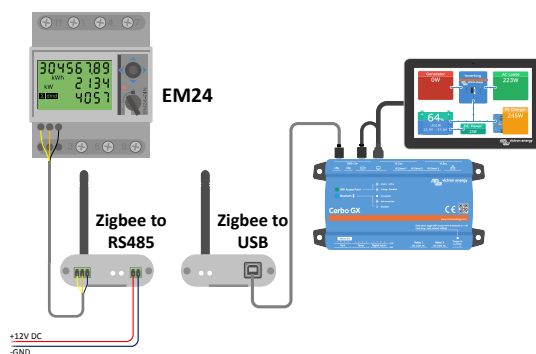
Energymeter draadloos Zigbee-verbinding met een Cerbo GX
