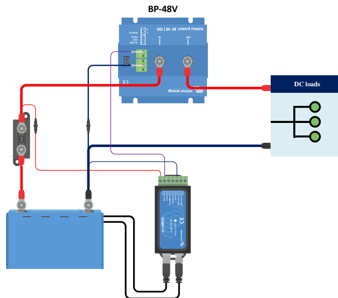
BatteryProtect gebruikt de belasting ontkoppelen van een smallBMS
