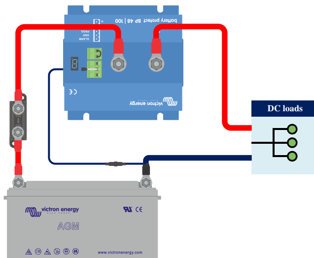
BatteryProtect in een eenvoudig systeem met draadlus tussen L en H-ingang (fabrieksstandaard)
