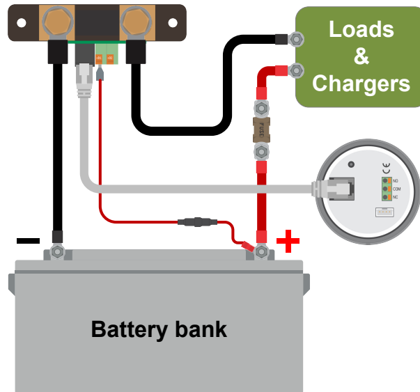
Installatie basis accubewaker.
