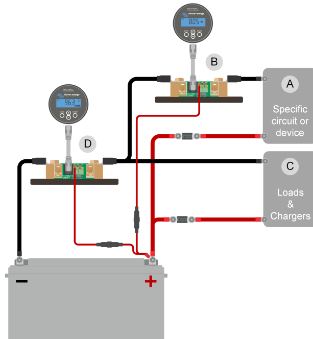
Bedravingsvoorbeeld van een systeem met een hoofd-accubewaker, samen met een accubewaker die opgezet werd als een DC-meter en bewaakt een specifiek apparaat of circuit. Eén accubewaker wordt gebruikt als een DC-meter (B) en de andere accubewaker wordt gebruikt als accubewaker (D).
