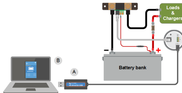
Voorbeeld van een VE.Direct-naar-USB-interface-verbinding tussen de accubewaker en een computer.
