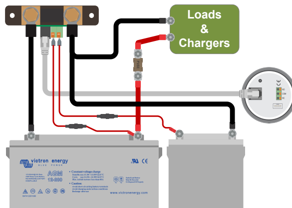
Accubewaker met bewaking reserve tweede accu.
