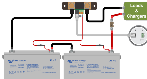
Accubewaker met reserve middelpuntbewaking.
