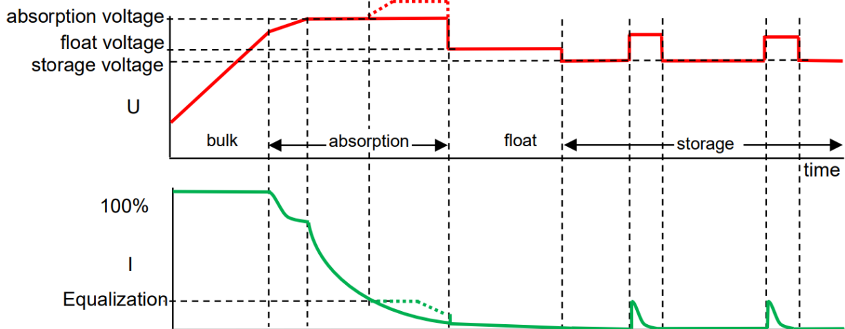
Abbildung 3 Spannung und Strom während verschiedener Zustände beim Laden der Batterie.
