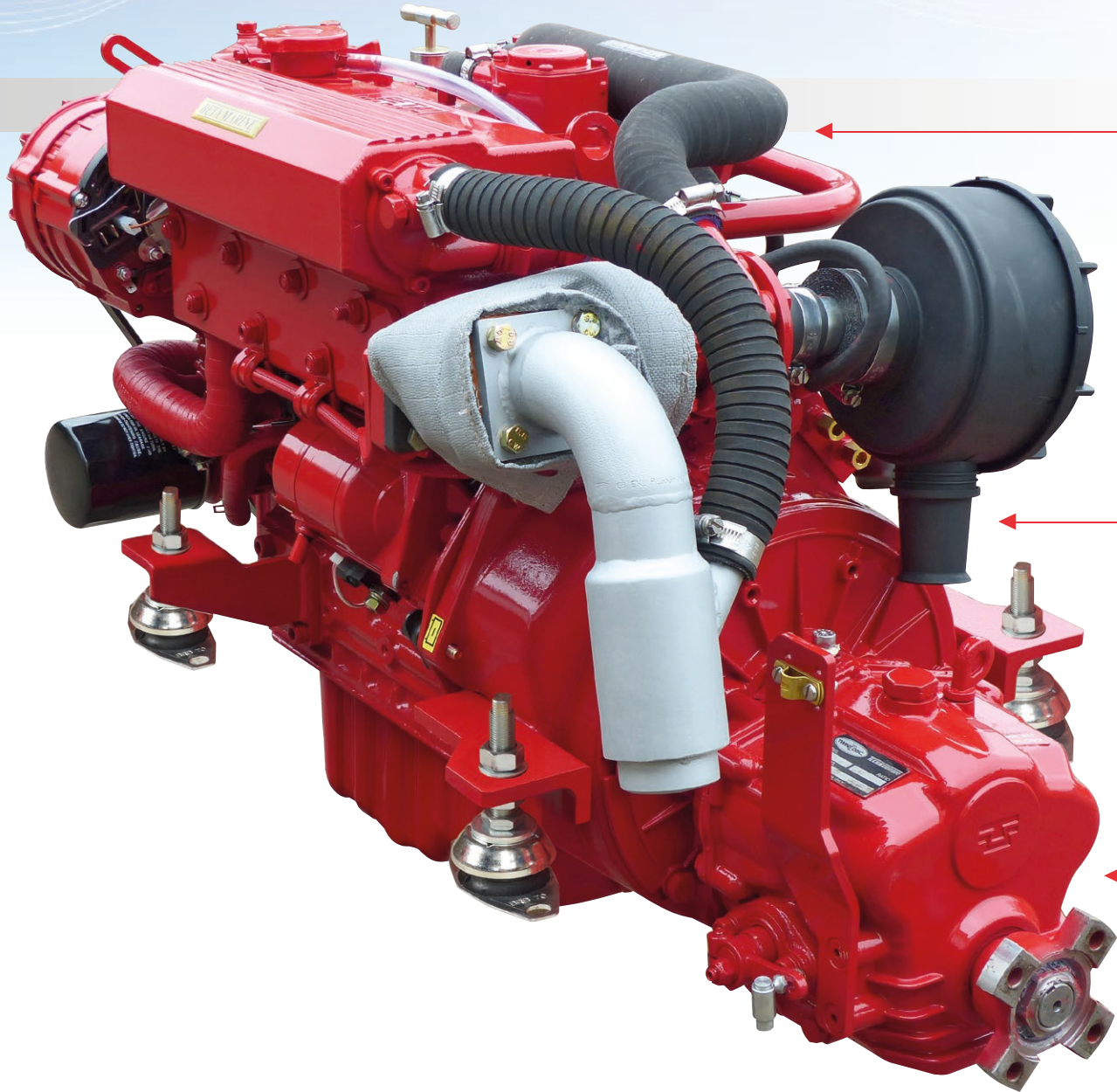
BETA 45T
